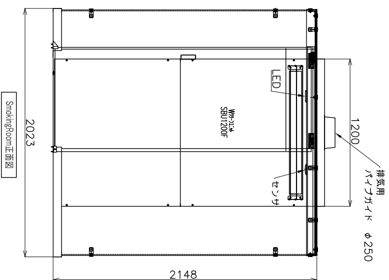
SmokingRoom 下辺平面図
